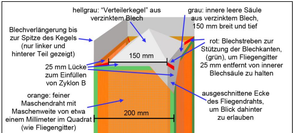
Abbildung 25: Schemazeichnung des oberen Teils der innersten Säule der Einwurfvorrichtung, wie sie anfangs von Kula am 11.6.1945 beschrieben wurde. (Rudolf 2020a, S. 155).
