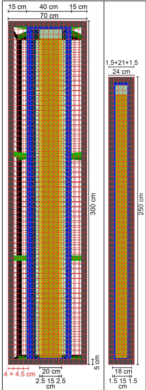
Abbildung 24a&b: Zeichnung der Zyklon-B-Einwurfssäule wie von Michal Kula am 11.6.1945 (links) bzw. beim Höß-Prozess beschrieben (rechts; Rudolf 2020a, S. 154).
