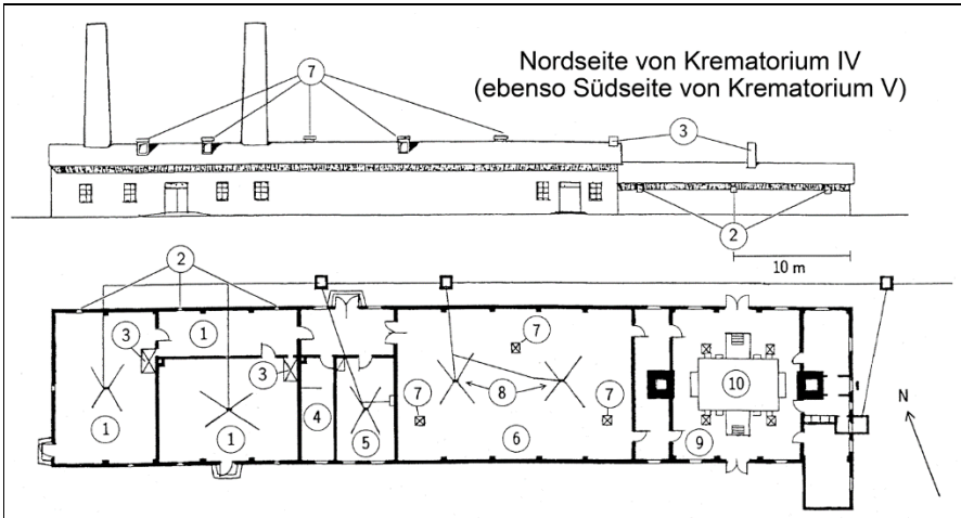
Abbildung 12: Nordseitenansicht und Grundriss von Krematorium IV bzw. V (spiegelbildlich) im Lager Auschwitz II/Birkenau (bereinigte Pläne, wie sie in Pressac 1989, S. 401 zu finden sind; aus Rudolf 2017a, S. 162) 1: Angebliche "Gaskammern"; 2: Angebliche Zyklon-B-Einwurfsluken; 3: Heizöfen; 4: Koksraum; 5: Arztraum; 6: Leichenhalle; 7: Lüftungskamine in Leichenhalle und Ofenraum – aber nicht in den "Gaskammern"; 8: Abflüsse; 9: Ofenraum; 10: Kremierungsöfen
