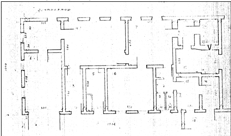
Dokument 3: Plan des Krematoriums von Sachsenhausen. Raum Nr. 2 (links oben) war die Gaskammer. GARF, 7021-104-3, S. 7.
