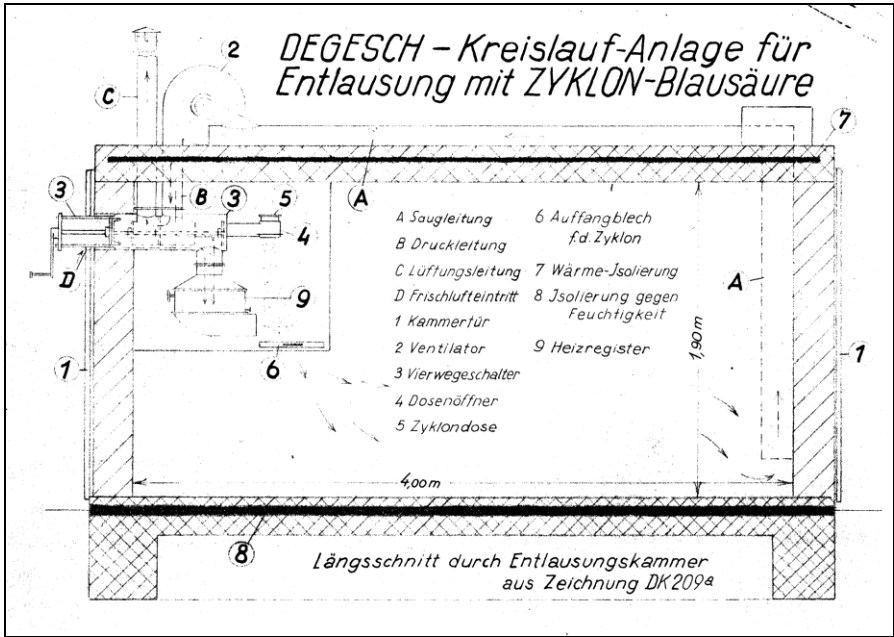
Dokument 2: Degesch-Kreislauf-Anlage für Entladung mit Zyklon Blausäure. APMM, VI, 9a, Bd. 2, S. 1-4.
