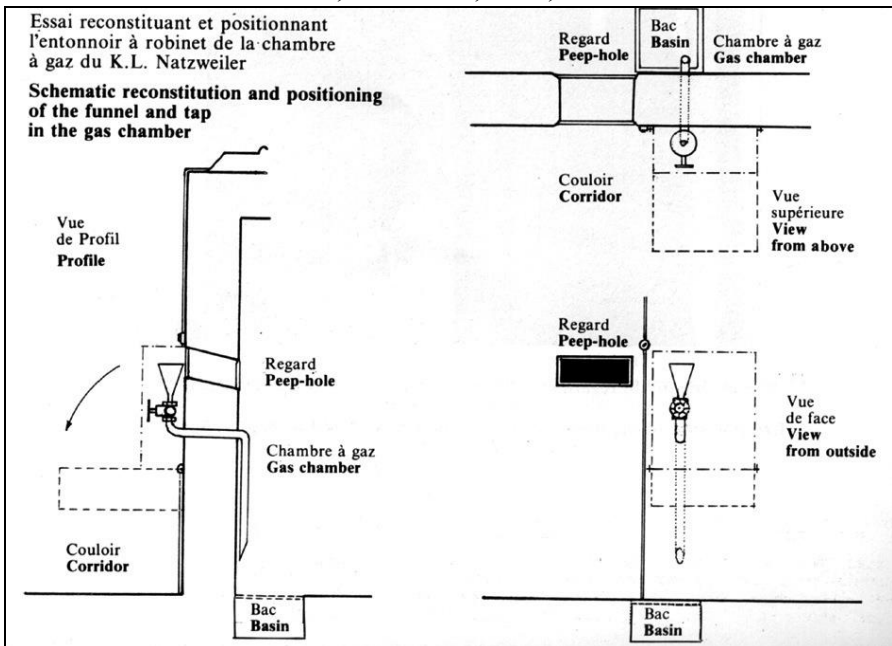
Dokument 7: Schemazeichnung der angebliche Einführungsrichtung der Gaskammer von Natzweiler-Struthof von J.-C. Pressac. Aus: ebenda, S. 66.
