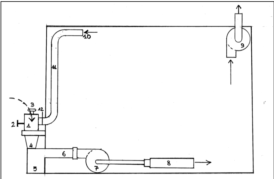
Dokument 5: Funktionsschema der technischen Einrichtung der Gaskammer von Sachsenhausen. © Carlo Mattogno.
