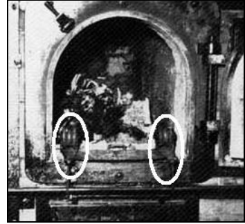
Abb. 3: Rollen vor der Muffeltür zur Einführung der Tragbahre (siehe weiße Ellipsen). 11
