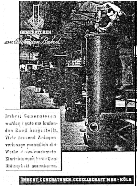
Abb. 132: Der Imbert-Generator war der meist verbreitete Holzgasgenerator des Dritten Reiches, hier in Massenproduktion „am laufenden Band“ im Werk Köln im Jahre 1943. (Motortechnische Zeitschrift, Nr. 6/7, 1943, S. 3A.)
