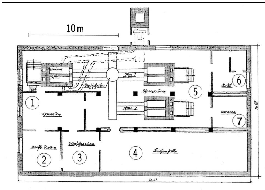
Abb. 104: Grundriss des Krematoriums I im Lager Auschwitz I/Stammlager im ursprünglichen Planungszustand. Die Leichenhalle soll später angeblich als Gaskammer benutzt worden sein. 1: Vorräum; 2: Aufbahrungsraum; 3: Waschraum; 4: Leichenhalle; 5: Ofenraum; 6: Koks; 7: Urnen
