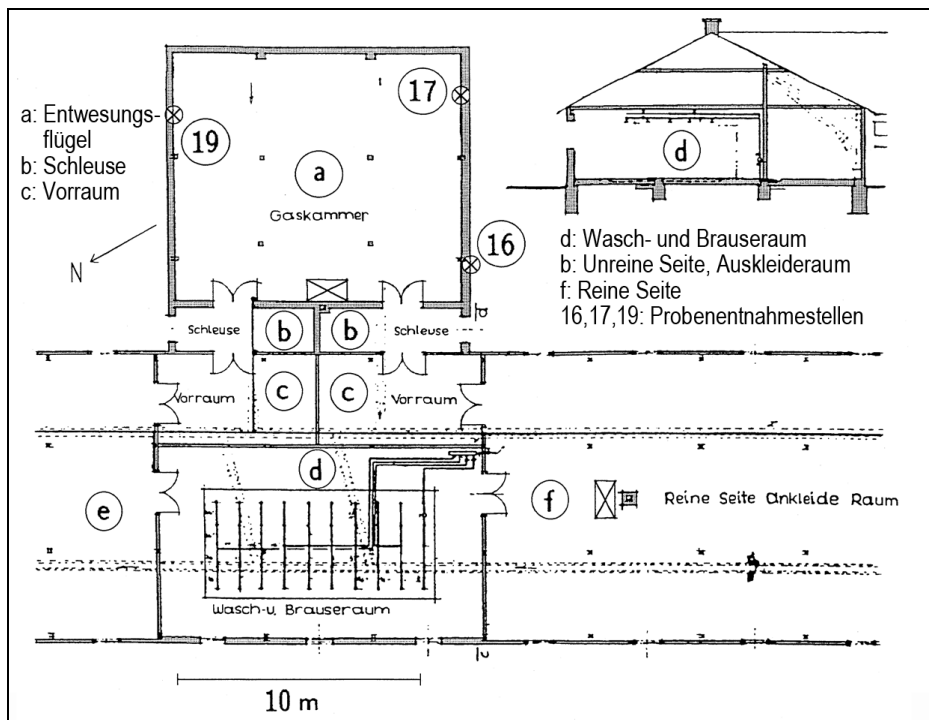
Abb. 115: Grundriss des HCN-Entwässerungstrakts der Bauwerke 5a vor dem Umbau (spiegelbildlich) und BW 5b bis heute. 203
